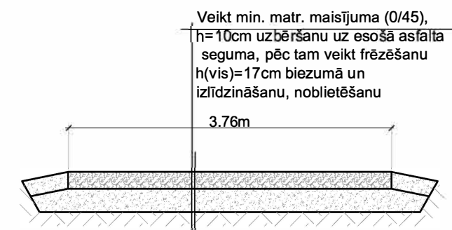
2 - 2 Piebraucamā laukuma šķērsgriezums M 1 : 50
